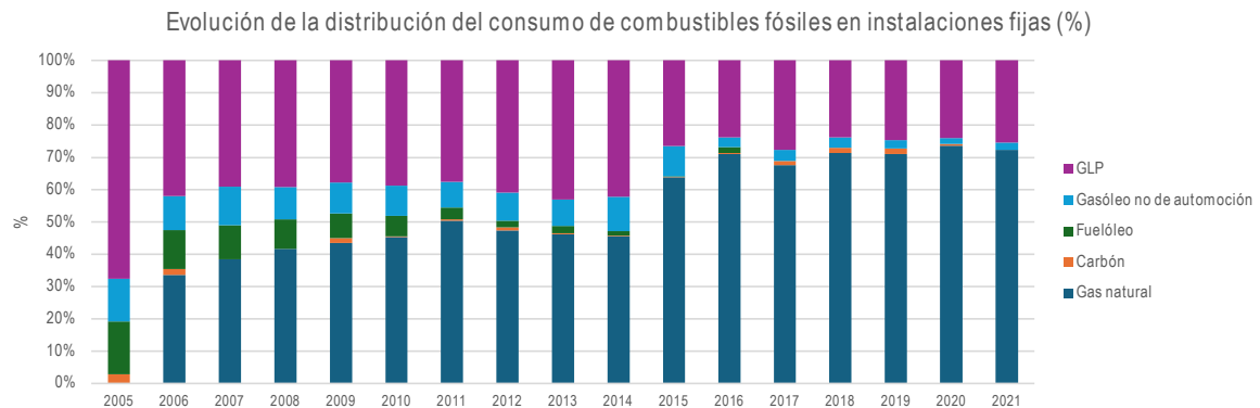
Figura 25. Evolución de la distribución del consumo de combustibles fósiles en las instalaciones fijas de 2005 a 2021. Fuente: Elaboración propia a partir de datos procedentes de la aplicación HCM de la Junta de Andalucía
