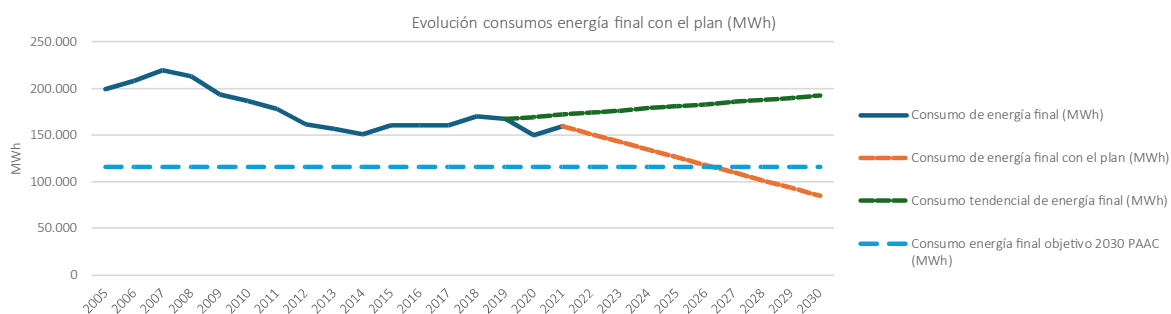
Figura 60. Evolución de los consumos de energía final esperadas en Castilla de la Cuesta con la aplicación del PMCC.
